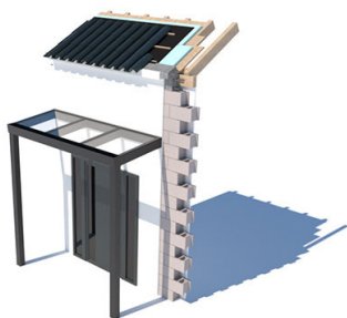
Zadaszenie drzwi wejściowych
